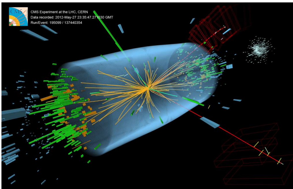
شکل ۲: رویداد ثبت شده توسط آشکارساز CMS در برخورد های پروتون-پروتون با انرژی مرکز جرم ۸ ترالکترونولت در سال ۲۰۱۲. این رویداد ویژگی های موردانتظار از واپاشی بوزون هیگز مدل استاندارد به یک جفت بوزون Z را نشان می دهد که یکی از آنها به یک جفت الکترون (خط های سبز با امتداد سبزرنگ قطورتر) و دیگری به یک جفت میونون (خط های قرمز) واپاشی کرده است. این رویداد همچنین می تواند ناشی از فرآیندهای شناخته شده پس زمینه در مدل استاندارد باشد.
