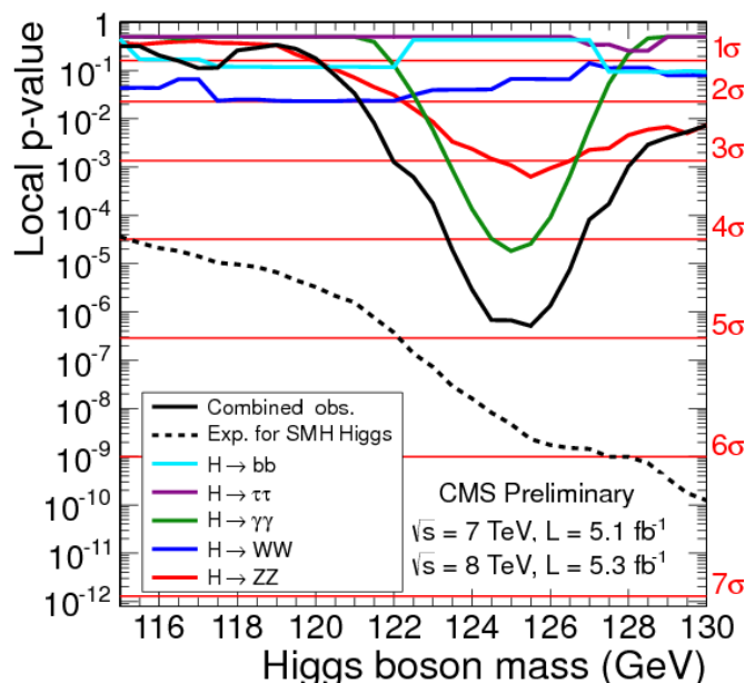
شکل ۵: احتمال موضعی (local P-Value) مشاهده شده از اینکه فرضیه «پس زمینه تنها» تعداد رویدادهایی یکسان یا بیش از آنچه در داده های CMS دیده شده بدست دهد، را به صورت تابعی از جرم هیگز مدل استاندارد در ۵ شاخه مورد مطالعه نشان می دهد. خط توپر سیاه احتمال موضعی ترکیبی برای تمامی شاخه ها می باشد.
