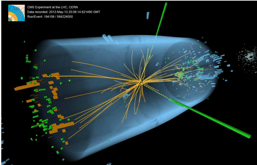
شکل ۱: رویداد ثبت شده توسط آشکارساز CMS در برخورد های پروتون-پروتون با انرژی مرکز جرم ۸ ترالکترونولت در سال ۲۰۱۲. این رویداد ویژگی های موردانتظار از واپاشی بوزون هیگز مدل استاندارد به یک جفت فوتون (خط چین های زرد و امتداد سبزرنگ قطور آنها) را نشان می دهد. این رویداد همچنین می تواند ناشی از فرآیندهای شناخته شده پس زمینه در مدل استاندارد باشد.
