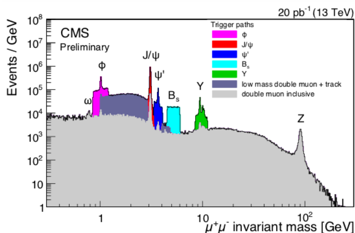
图 2: 13 TeV 能量下 \mu 子对的不变质量谱
