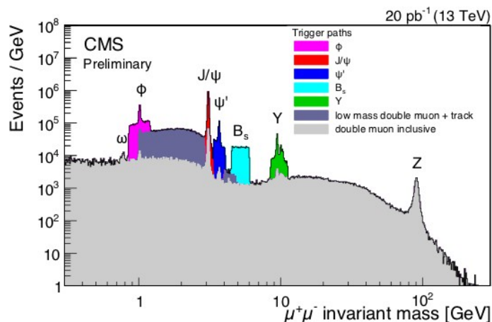
Figure 2: Rozkład masy niezmienniczej par mionów zarejestrowanych przy energii 13 TeV.
